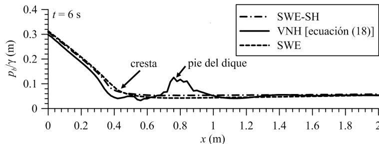
Figura 6 | Comparativa de las predicciones de presiones dinámicas en el fondo por los modelos SWE, SWE-SH y VNH para el test 55 de Schomcker (2011) en el instante t = 6 s.
